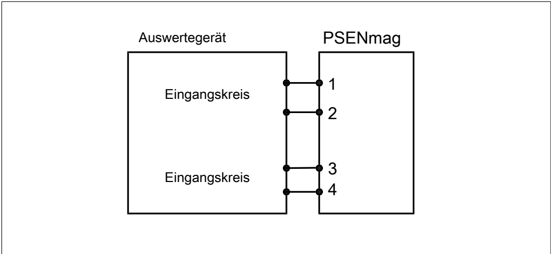
Abb.: Zweikanaliger Anschluss des PSEN ma1.4p-50 an den Eingangskreisen eines Auswertegeräts
