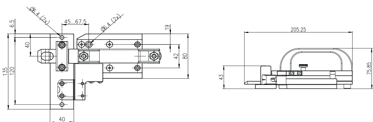
Fig. 7: Montage und Abmessungen PSEN b mit PSENcode oder PSENmag, using a left-hinged gate as an example/Montage et dimensions du PSEN b avec PSENcode ou PSENmag dans l'exemple avec protecteur ouvert à gauche
