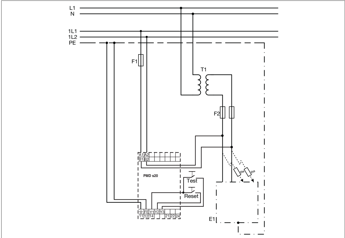
► Anwendungsschaltung DC
