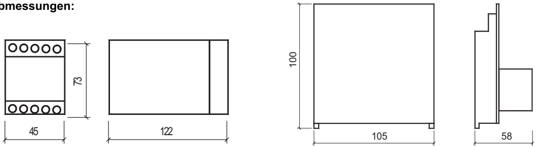
Gehäuseausführung
