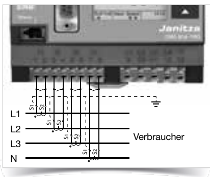
Abb.: Strommessung über Stromwandler
