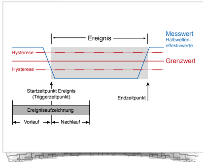
Abb.: Die Ereignisaufzeichnung beinhaltet einen Mittelwert, einen Minimum- bzw. Maximumwert, einen Start- und einen Endzeitpunkt.
