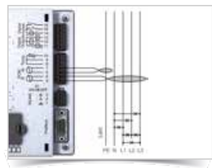
Abb.: Anschlussbeispiel Differenzstrommessung und PE über Stromwandler
