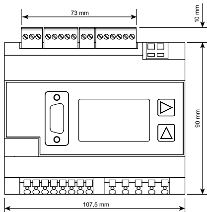
Vorderansicht
