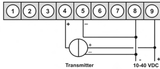
M3 in Verbindung mit einem 3-Leiter-Sensor 0/4-20 mA
