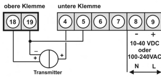
3-Leiter-Sensor 0-20 mA
