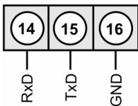
Schnittstelle RS232 (Modbus Protokoll)
