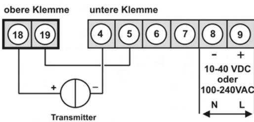
2-Leiter-Sensor 4-20 mA
