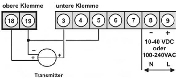
3-Leiter-Sensor 0-10 V
