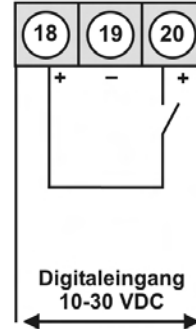
M3 mit Digitaleingang in Verbindung mit 24 VDC Geberversorgung
