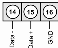
Schnittstelle RS485 (Modbus Protokoll)
