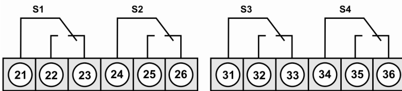
Relais 1 und 2
