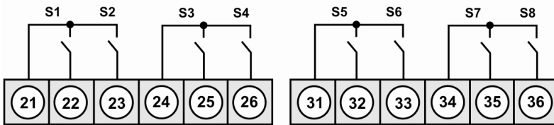
8 PhotoMos-Ausgänge
